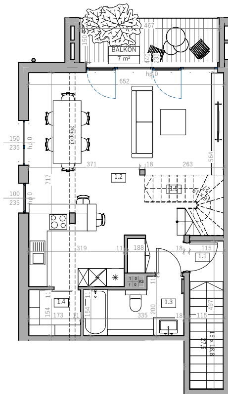
RZUT PODDASZA
