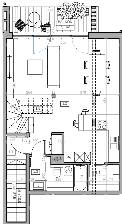
RZUT PODDASZA
